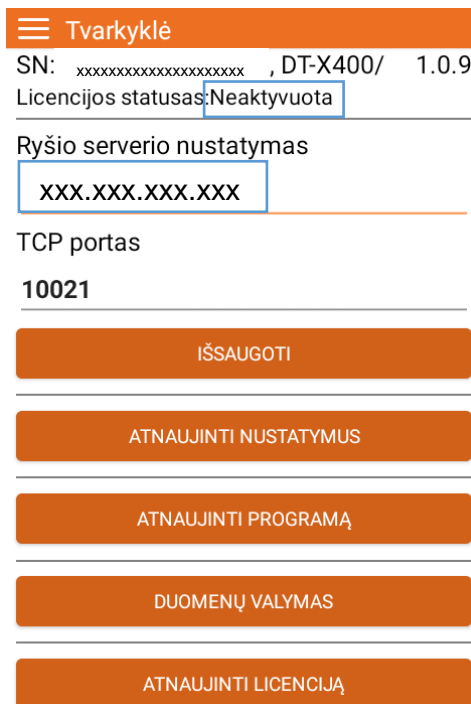
pav. 3 Tvarkyklės nustatymai
